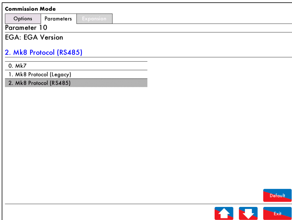
Figure 2.1.1 ii: Parameter 10 on the Mk8 or Mini Mk8 MM
